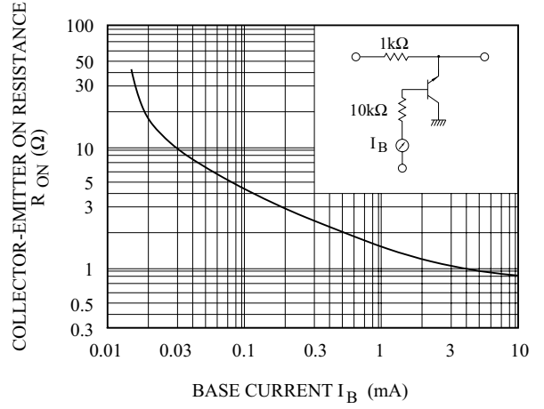
R_{ON} - I_B
